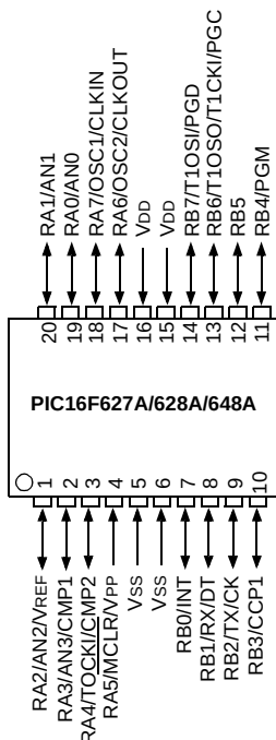
SSOP
